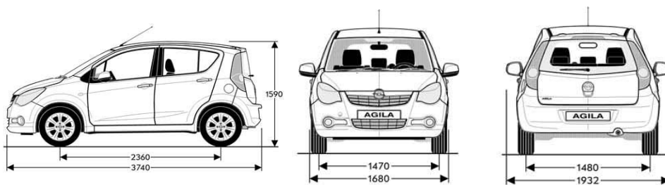
Dimensions en mm
